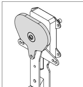
Manetta 'Pull'
