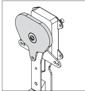
‚Zug‘-Hebel
