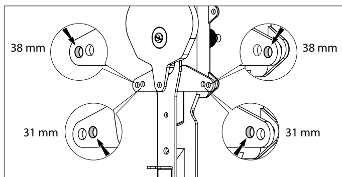
Corsa del cavo della scatola del cambio
