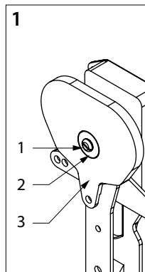
‚Zug‘-Hebel
