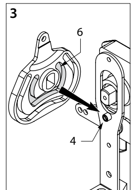
‚Schub‘-Hebel
